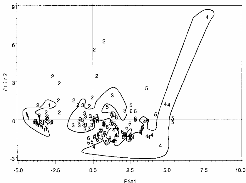
Figura 6: Cruzamento dos componentes principais 1 e 2, com distribuição espacial e temporal dos pontos de coleta.
