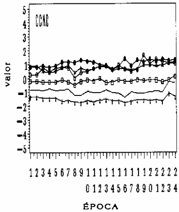
3: Distribuição temporal de variáveis. As escalas são apresentadas na forma padronizada 'Z', considerando 24 meses (03/96 a 03/98, exceto 01/97) numerados de 1 a 24, em 6 locais: 1. nascente da mata (—), 2. nascente do sistema (—|—), 3. açude do sistema (—), 4. água corrente cavalariça (—●—), 5. açude da colônia (—○—) e 6. água corrente na foz (—X—).
