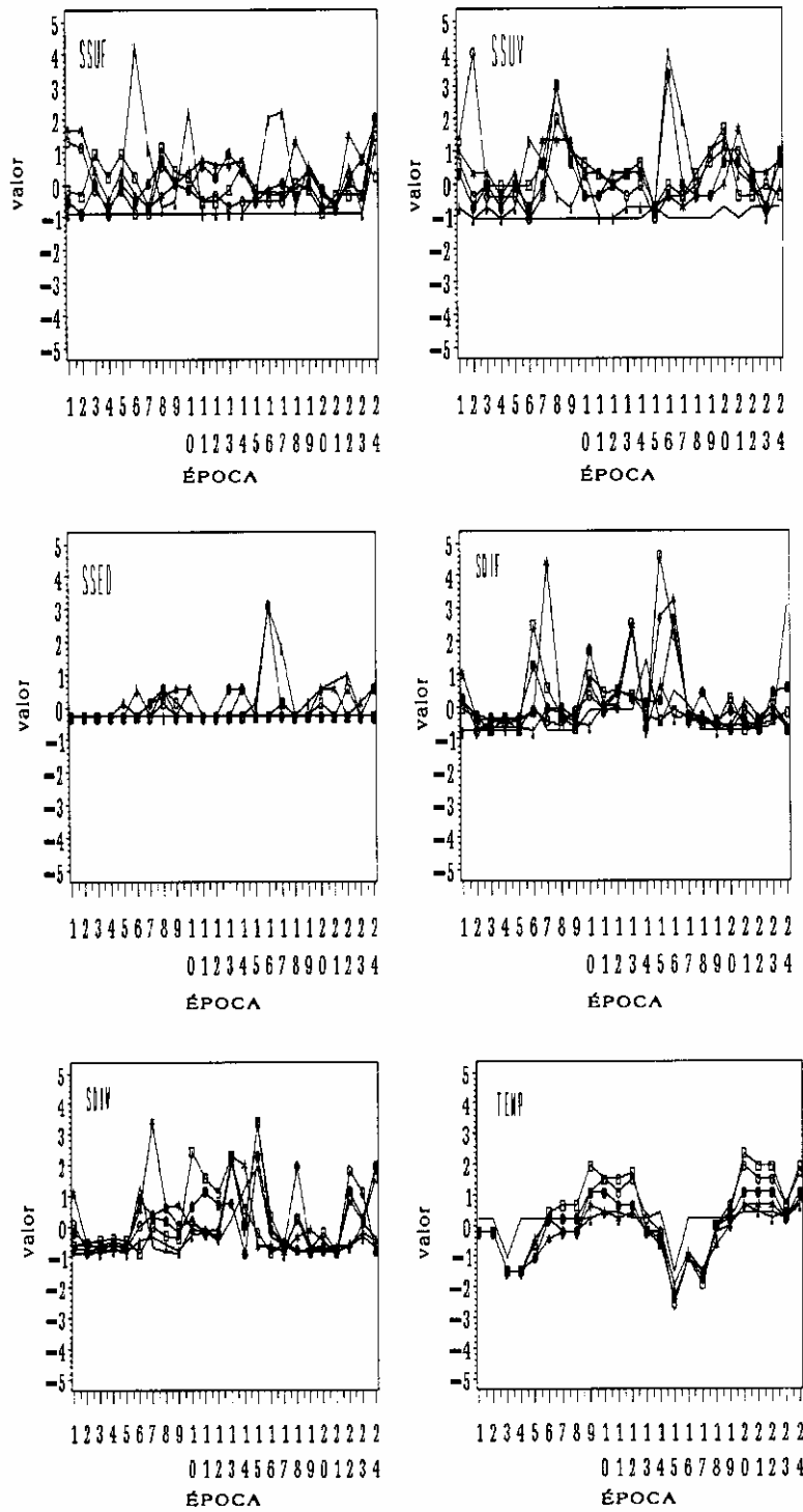
Figura 5: Distribuição temporal de variáveis. As escalas são apresentadas na forma padronizada 'z', considerando 24 meses (03/96 a 03/98, exceto 01/97) numerados de 1 a 24, em 6 locais: 1. nascente da mata (—), 2. nascente do sistema (—|—), 3. açude do sistema (—), 4. água corrente cavalariça (—●—), 5. açude da colônia (—○—) e 6. água corrente na foz (—✕—).
