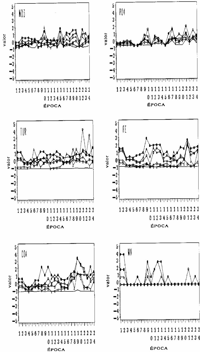
Figura 4: Distribuição temporal de variáveis. As escalas são apresentadas na forma padronizada 'z', considerando 24 meses (03/96 a 03/98, exceto 01/97) numerados de 1 a 24, em 6 locais: 1. nascente da mata (—), 2. nascente do sistema (—□—), 3. açude do sistema (—△—), 4. água corrente cavalariça (—●—), 5. açude da colônia (—◇—) e 6. água corrente na foz (—×—).
