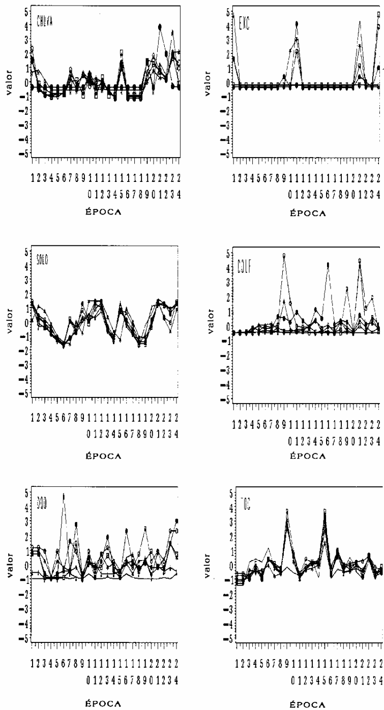
Figura 2: Distribuição temporal de variáveis. As escalas são apresentadas na forma padronizada 'zi', considerando 24 meses (03/96 a 03/98, exceto 01/97) numerados de 1 a 24, em 6 locais: 1. nascente da mata (—), 2. nascente do sistema (—|), 3. açude do sistema (— —), 4. água corrente cavalariça (—●—), 5. açude da colônia (—○—) e 6. água corrente na foz (—X—).
