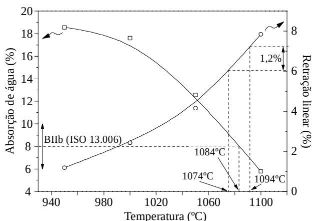
Figura 1. Curvas de gresificação de massas utilizadas industrialmente para a fabricação de vários produtos cerâmicos.
