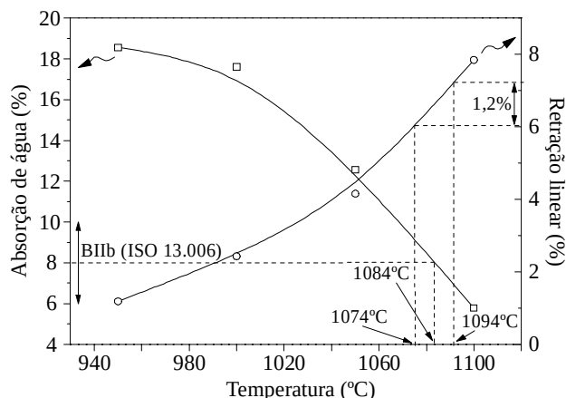
Figura 2. Curva de gresificação de uma massa industrial utilizada na fabricação de pisos por via seca.
