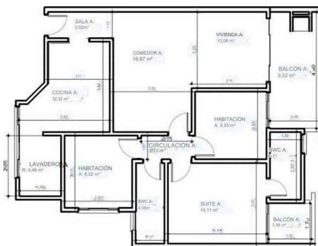
Cifra 1: plano bajo del departamento tipo.
