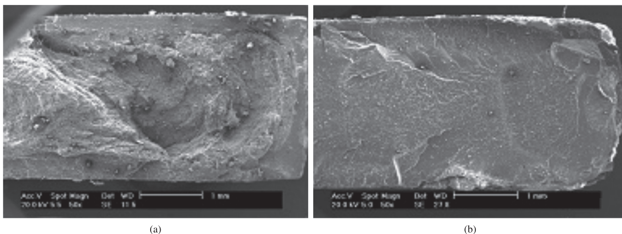
Figura 8. Micrografias da superfície de fratura de corpos-de-prova de impacto (região próxima a solicitação) expostos por 15 semanas para as blendas a) 70/30 v e b) 90/1 v.
