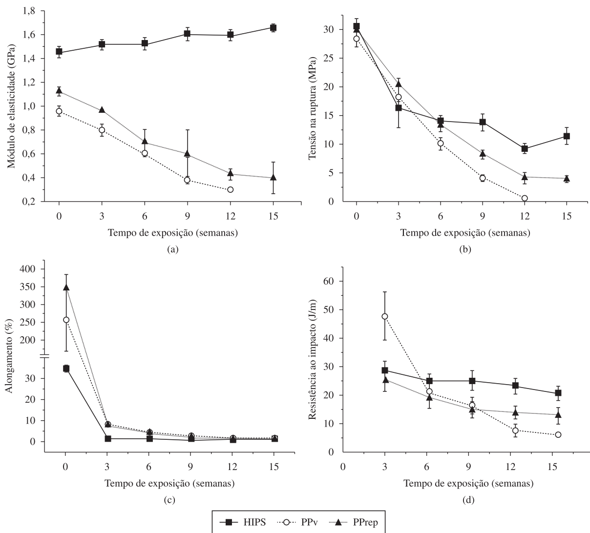
Figura 1. Efeito do tempo de exposição nos valores médios do: a) Módulo de Elasticidade, b) tensão na ruptura, c) alongamento máximo, e d) resistência ao impacto para o HIPS, PPv e PPp. Os dados para o PPp e HIPS já foram apresentados [21] e são reportados aqui somente para fim de comparação.
