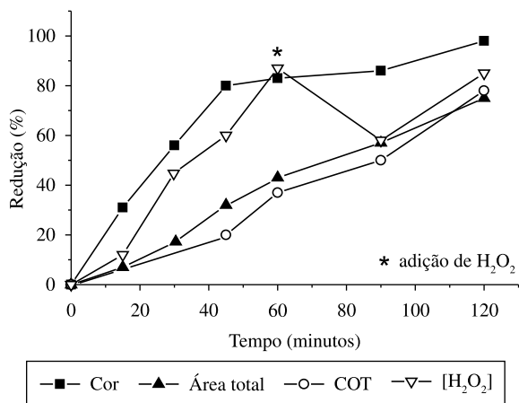
Figura 5. Acompanhamento da degradação do corante Azul QR 19 em solução ( 50 \text{ mg.L}^{-1} ) pelo processo foto-Fenton com luz solar, na temperatura ambiente. (Variáveis: redução da cor; da área espectral total; do carbono orgânico total e da concentração de peróxido de hidrogênio).
