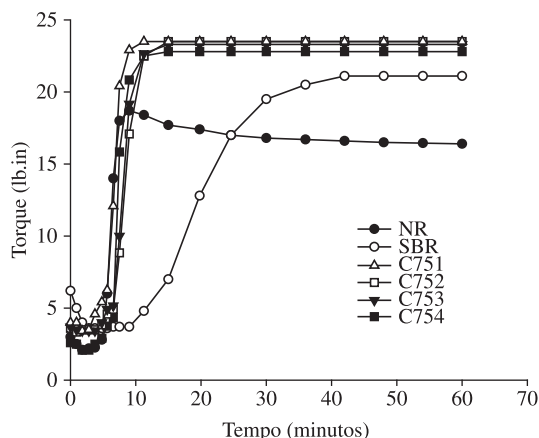
Figura 2. Curvas reométricas de misturas 75:25 NR/SBR.
