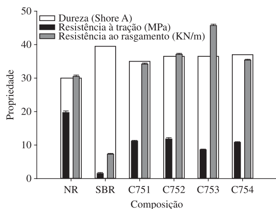
Figura 1. Propriedades mecânicas de misturas 75:25 NR/SBR.
