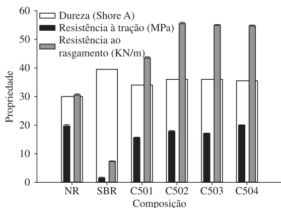
Figura 3. Propriedades mecânicas das misturas 50:50 NR/SBR.
