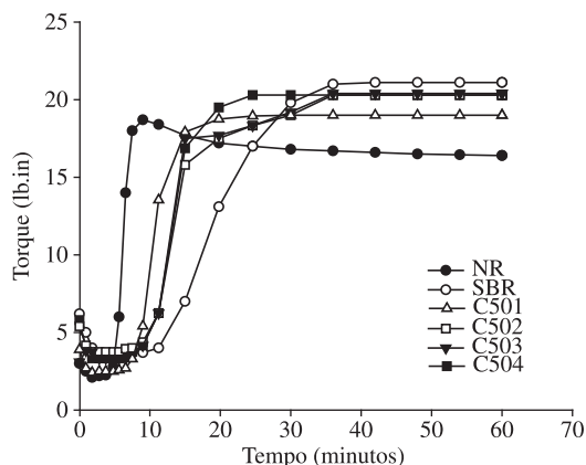
Figura 4. Curvas reométricas de misturas 50:50 NR/SBR.
