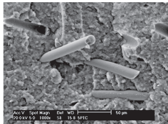
Figura 6. Micrografias eletrônicas de varredura dos compósitos com 5% de fibra picada 5PSC (em aumento de 500x) e 5PTC (em aumento de 1.000x).
