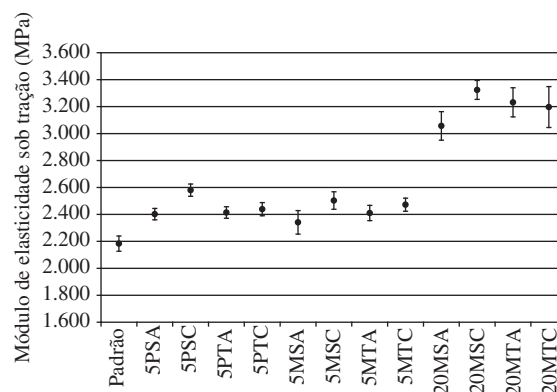
Figura 4. Módulos elásticos sob tração dos compósitos preparados.
