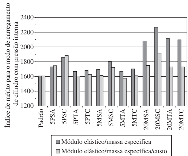
Figura 10. Índice de mérito para modo de carregamento de cilindro com pressão interna.
