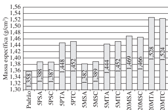
Figura 3. Massas específicas dos compósitos preparados.
