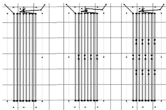
Figura 10. Desenho CAD das amostras dos modelos 11, 12 e 23.
