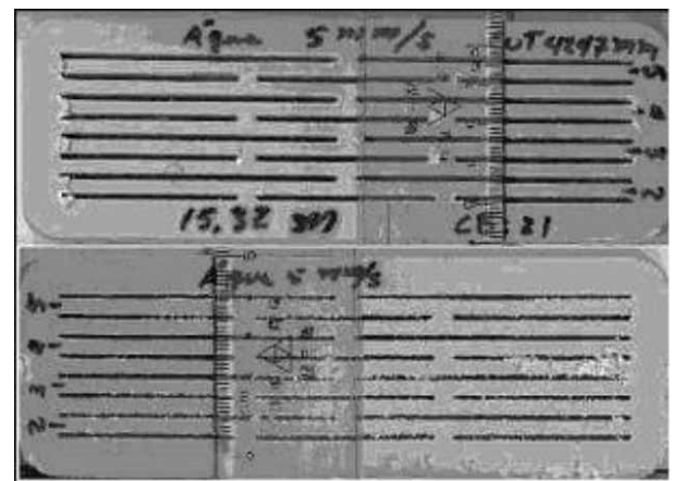
Figura 9. Mostrando QW, corte com água pura. Acima entrada e abaixo saída do jato.
