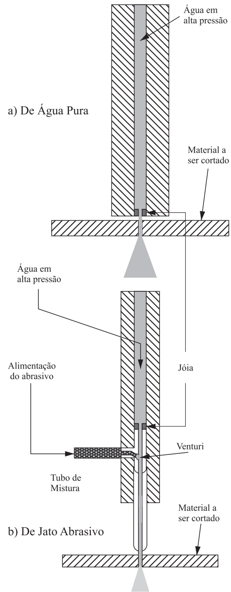
Figura 1. Tipos de bocais de corte
