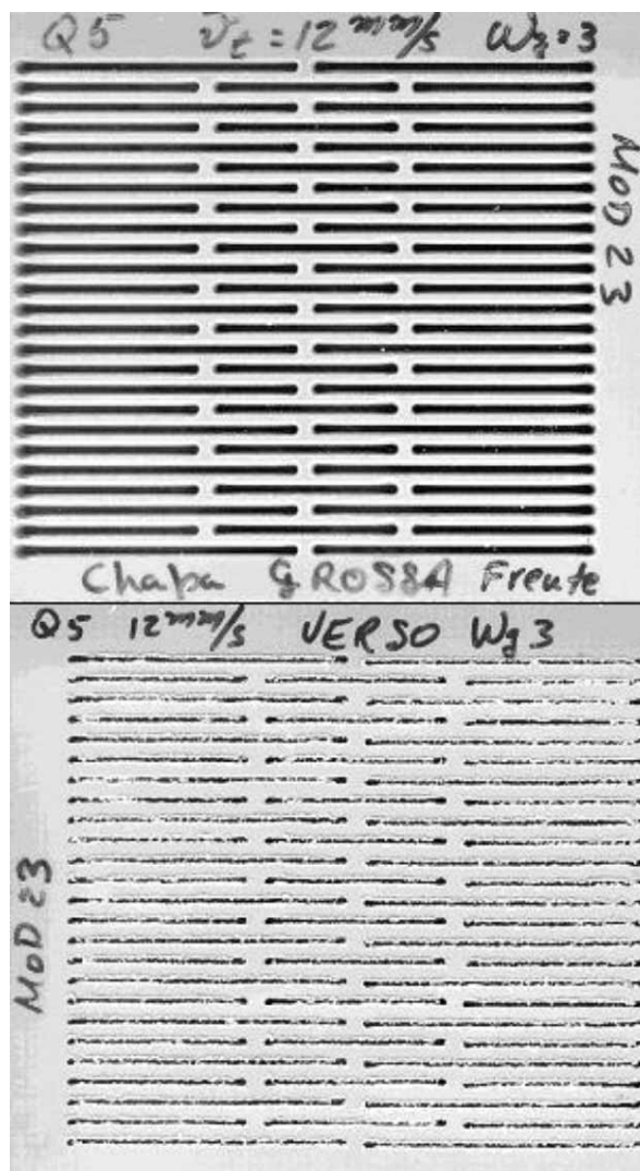
Figura 6 – Fotografias dos ensaios realizados nas qualidades Q5.
