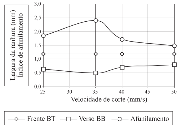
Figura 12. Índices de afunilamento no modelo 23
