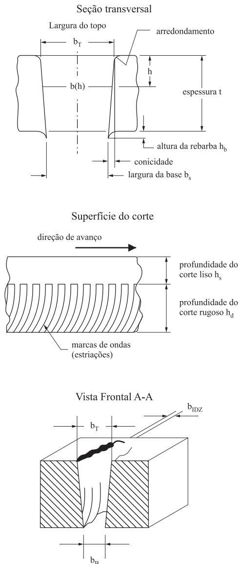
Figura 2. Elementos de sulcos gerados por jatos abrasivos.
