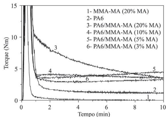
Figura 3. Misturas PA6/MMA-MA (90/10%).
