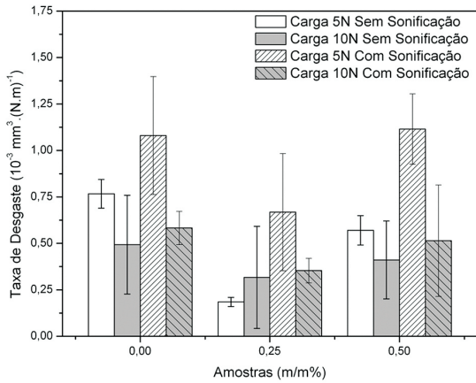
Figura 5. Taxa de desgaste dos nanocompósitos produzidos.
