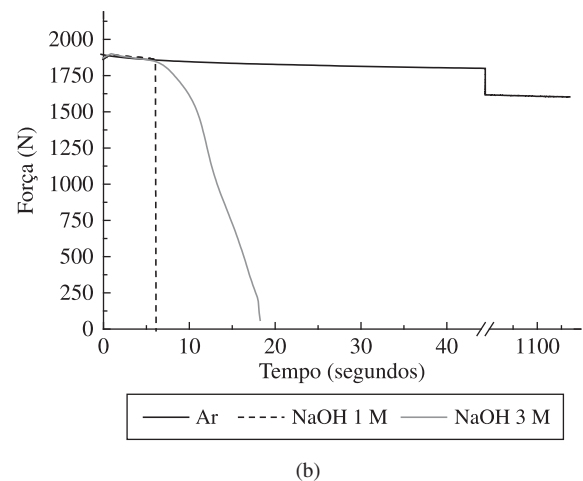
Figura 12. Curvas de relaxação de tensão do PET nas cargas de a) 1000 N; e b) 1900.
